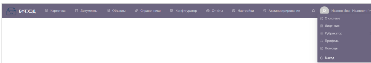
Рисунок 42 – Завершение работы
